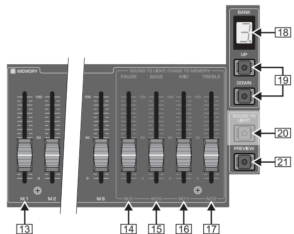
Abb. 2.3: Die B MEMORY-Sektion
