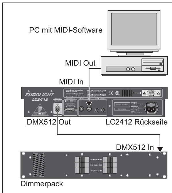
Abb. 7.4: MIDI-Verkabelung
