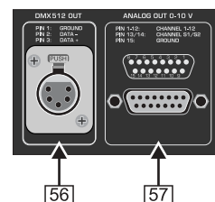
Abb. 2.9: Der digitale und der analoge Ausgang
