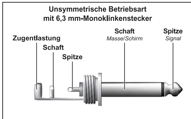
Abb. 9.2: Monoklinkenstecker für Audiosignal
