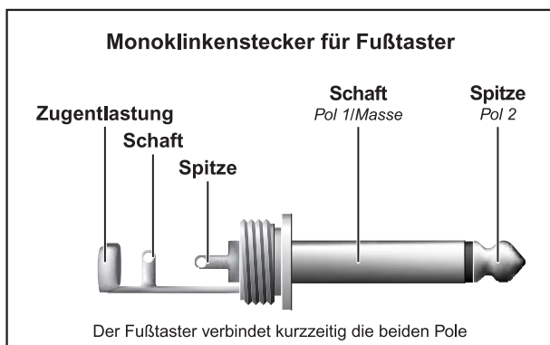
Abb. 9.3: Beschaltung des Fußtastersteckers
