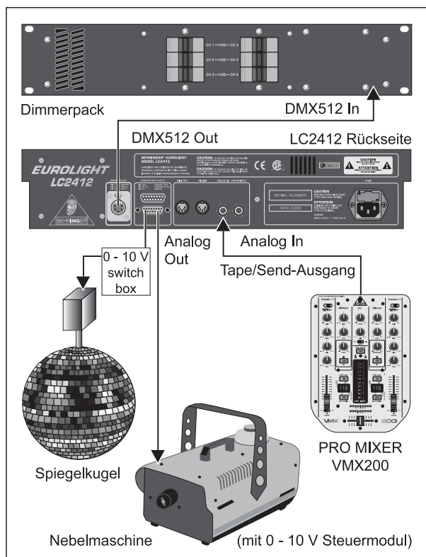
Abb. 8.1: Standardverkabelung an Dimmer mit analoger und/oder digitaler Steuerung
