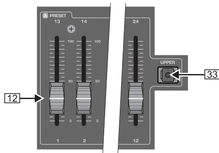
Abb. 2.2: Die A PRESET-Sektion (Ausschnitt)
