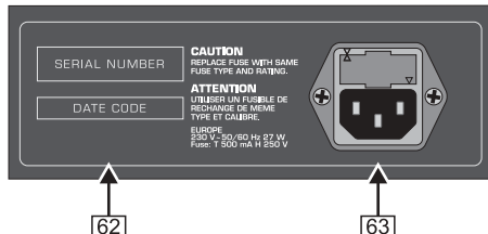
Abb. 2.11: Seriennummer und Netzanschluss
