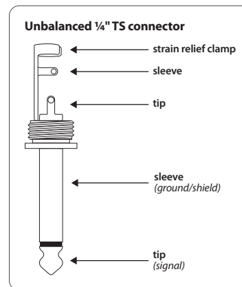
Abb. 5.2: 6,3-mm-Monoklinkenstecker
