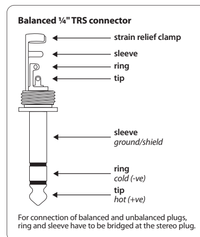
Abb. 5.3: 6,3-mm-Stereoklinkenstecker
